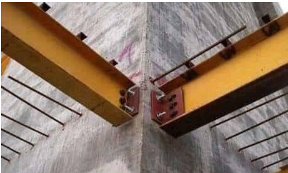
Ukážka uchytenia oceloveho nosnika do kotviacej platne v betone
