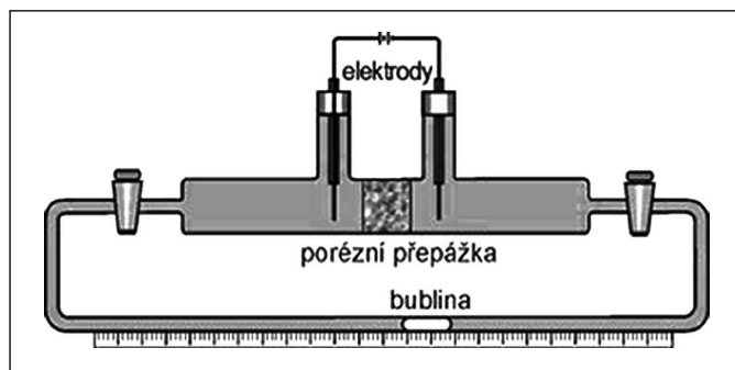
Měření elektroosmózy
